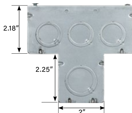
4-11/16" T Box
